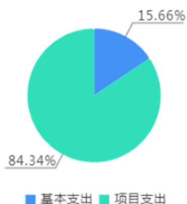
支出结构图
